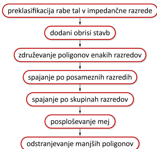
Slika 65: Postopek posploševanja karte dejanske rabe zemljišč MKGP v karto akustične impedanace.
