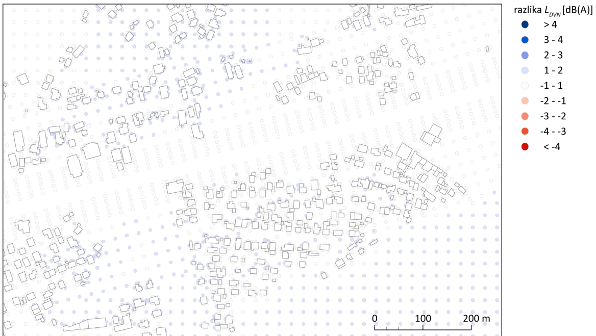
Slika 109: Karta razlik v ravni jakosti zvoka med referenčnim izračunom in izračunom z akustično impedanco, pridobljeno iz karte rabe tal oziroma pokrovnosti Corine.
