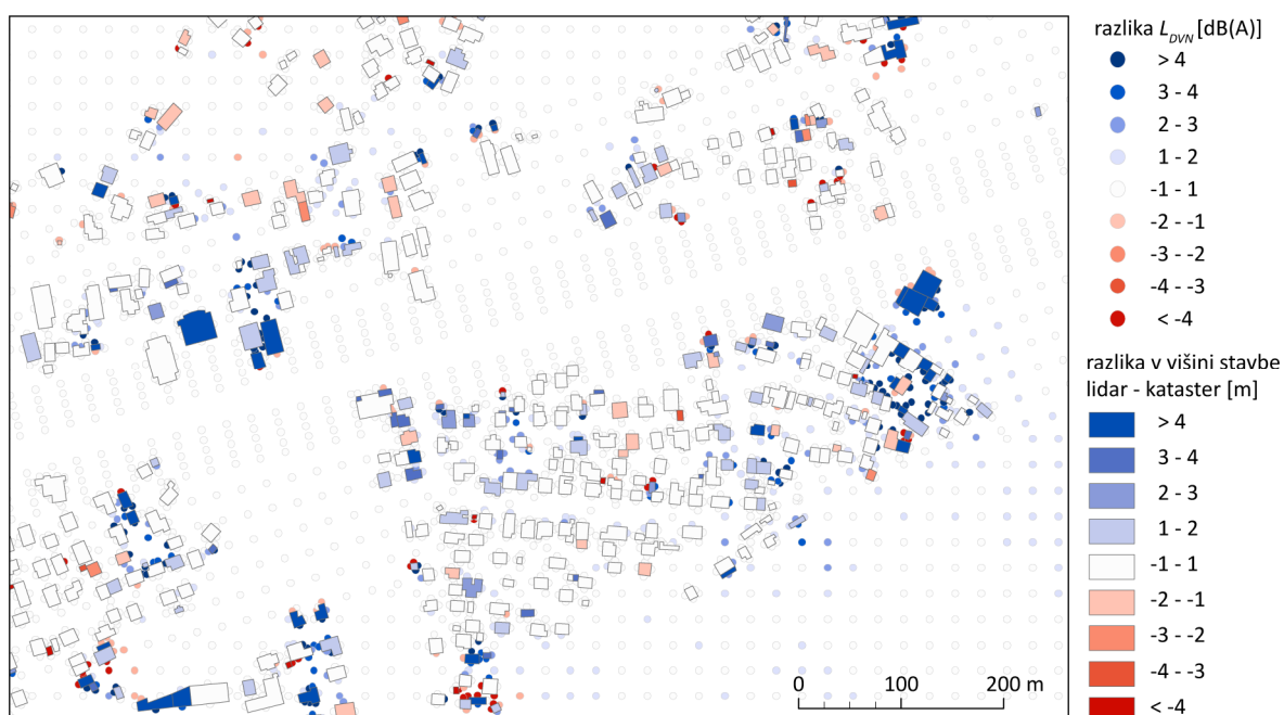
Slika 102: Karta razlik v ravni jakosti zvoka med referenčnim izračunom in izračunom z višinami slemena stavb iz katastra. V barvni lestvici so prikazane tudi razlike v višinah stavb med podatki laserskega skeniranja in katastrom stavb.
