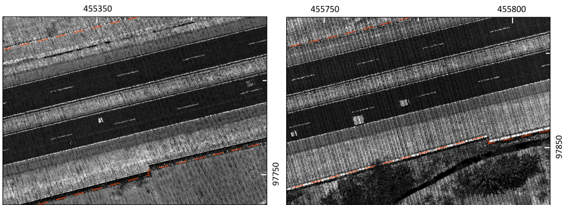
Slika 38: Slike intenzitete z nakazanima protihrupnima pregradama (črtkano blede rdeče). Južna pregrada na sliki desno odstopa od slike intenzitete, ker je pregrada nagnjena in vrh slabše odbija infrardeči laserski žarek od spodnjega dela, kar je ravno obratno, kot na sliki levo. Slika 39 prikazuje trirazsežni pogled obeh območij
