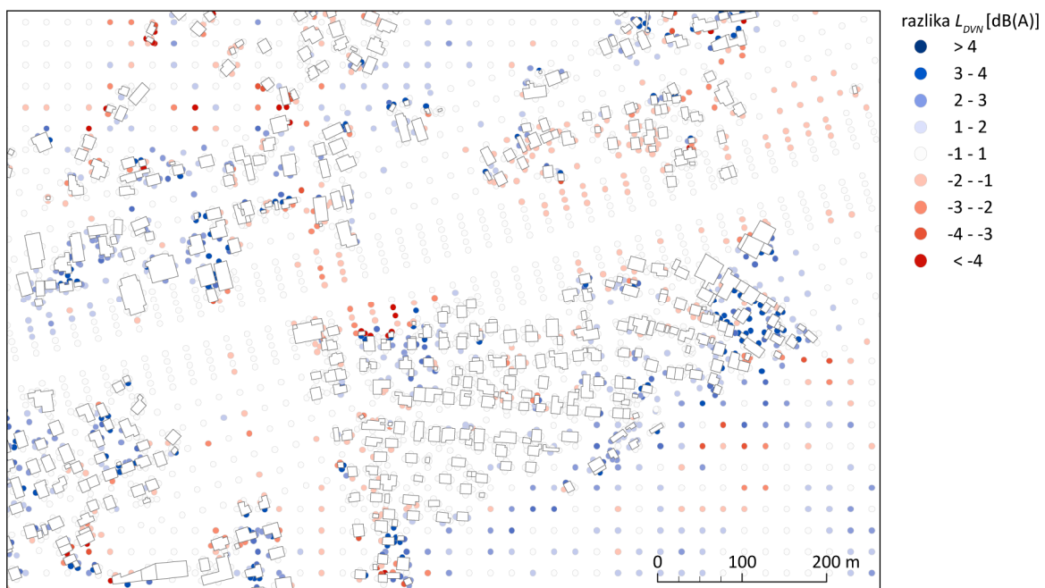
Slika 112: Karta razlik v ravni jakosti zvoka med referenčnim izračunom in izračunom s podatki GURS in brez upoštevanje impedance.
