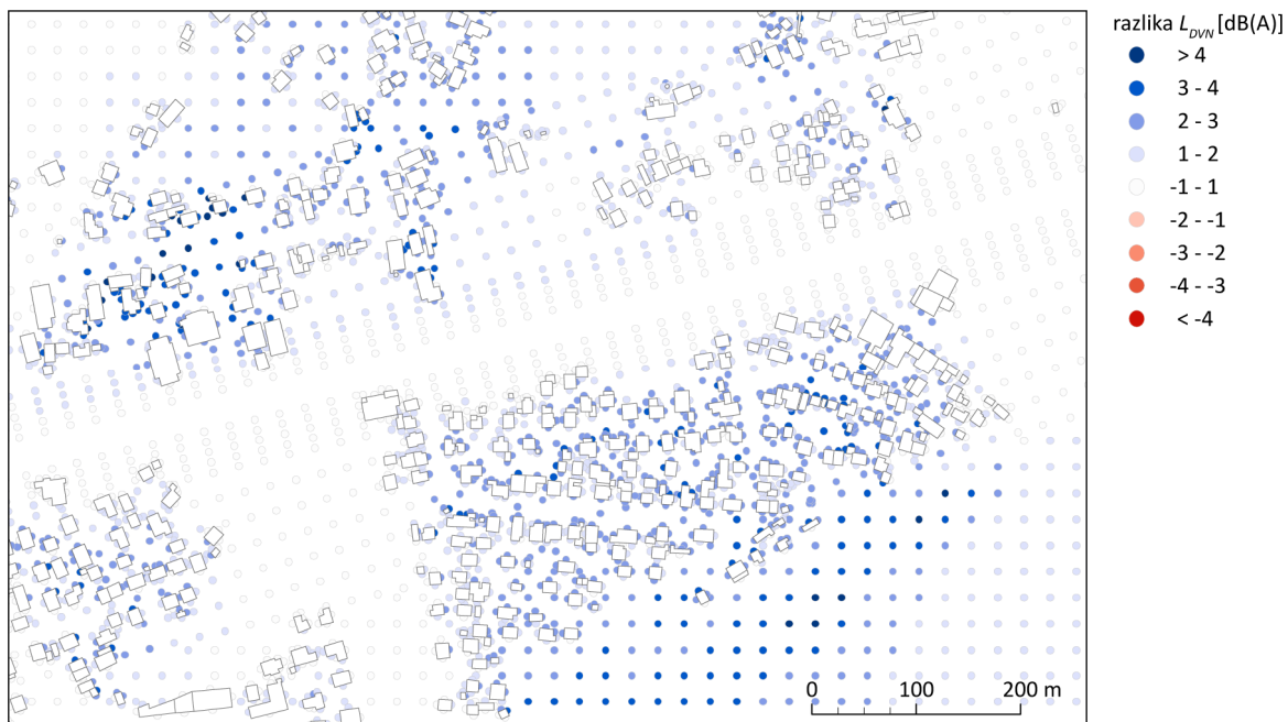
Slika 108: Karta razlik v ravni jakosti zvoka med referenčnim izračunom in izračunom z akustično impedanco, pridobljeno iz karte rabe tal oziroma pokrovnosti MKGP.
