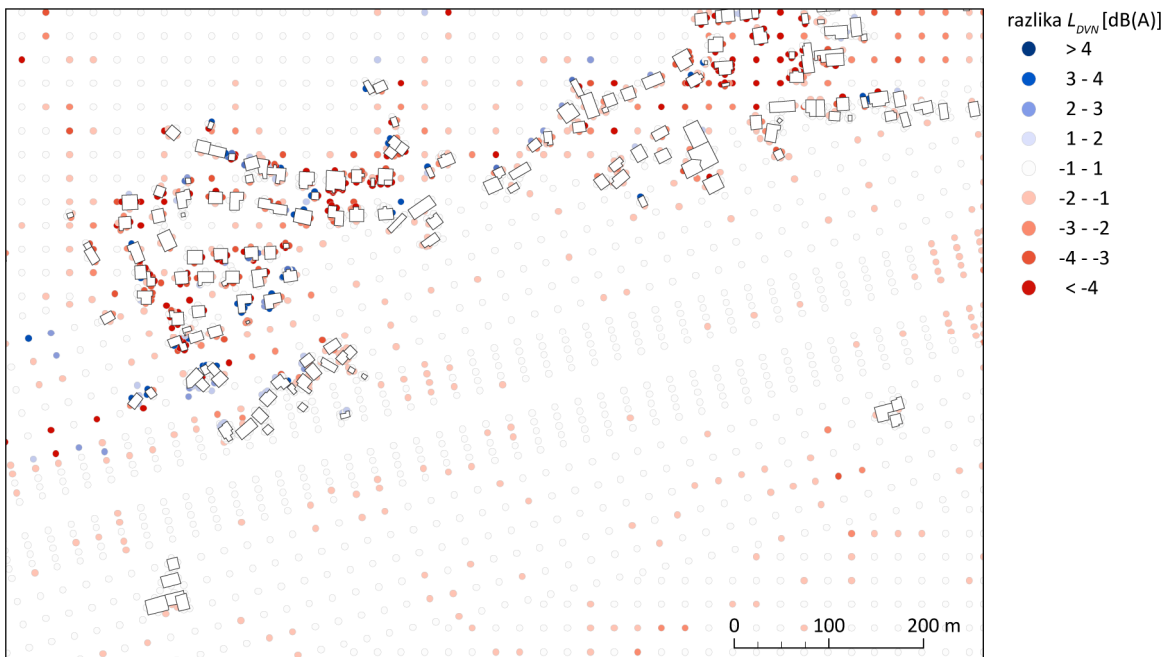
Slika 114: Karta razlik v ravni jakosti zvoka med referenčnim izračunom in izračunom s podatki GURS za ožje študijsko območje O1.
