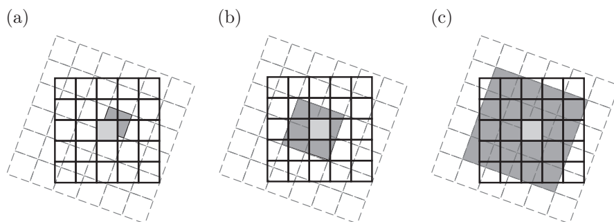
Slika 15.4: Interpolacija novih vrednosti pri prevzorčenju z metodo najbližjega sosa (a), z bilinearno interpolacijo (b) in s kubično konvolucijo (c). Vrednost v transformirani podobi (polna mreža) dobimo iz ene ali več vrednosti v prvotni (črtkano).
