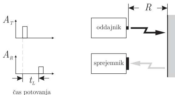
Slika 10.2: Lidar določa razdaljo med senzorjem in površjem z merjenjem časa potovanja valovanja.
