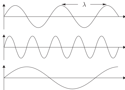
Slika 3.2: Valovanje opišemo z amplitudo, frekvenco in valovno dolžino. Srednji grafikon prikazuje visoko frekvenco oziroma majhno valovno dolžino, spodnji pa nizko frekvenco oziroma veliko valovno dolžino.
