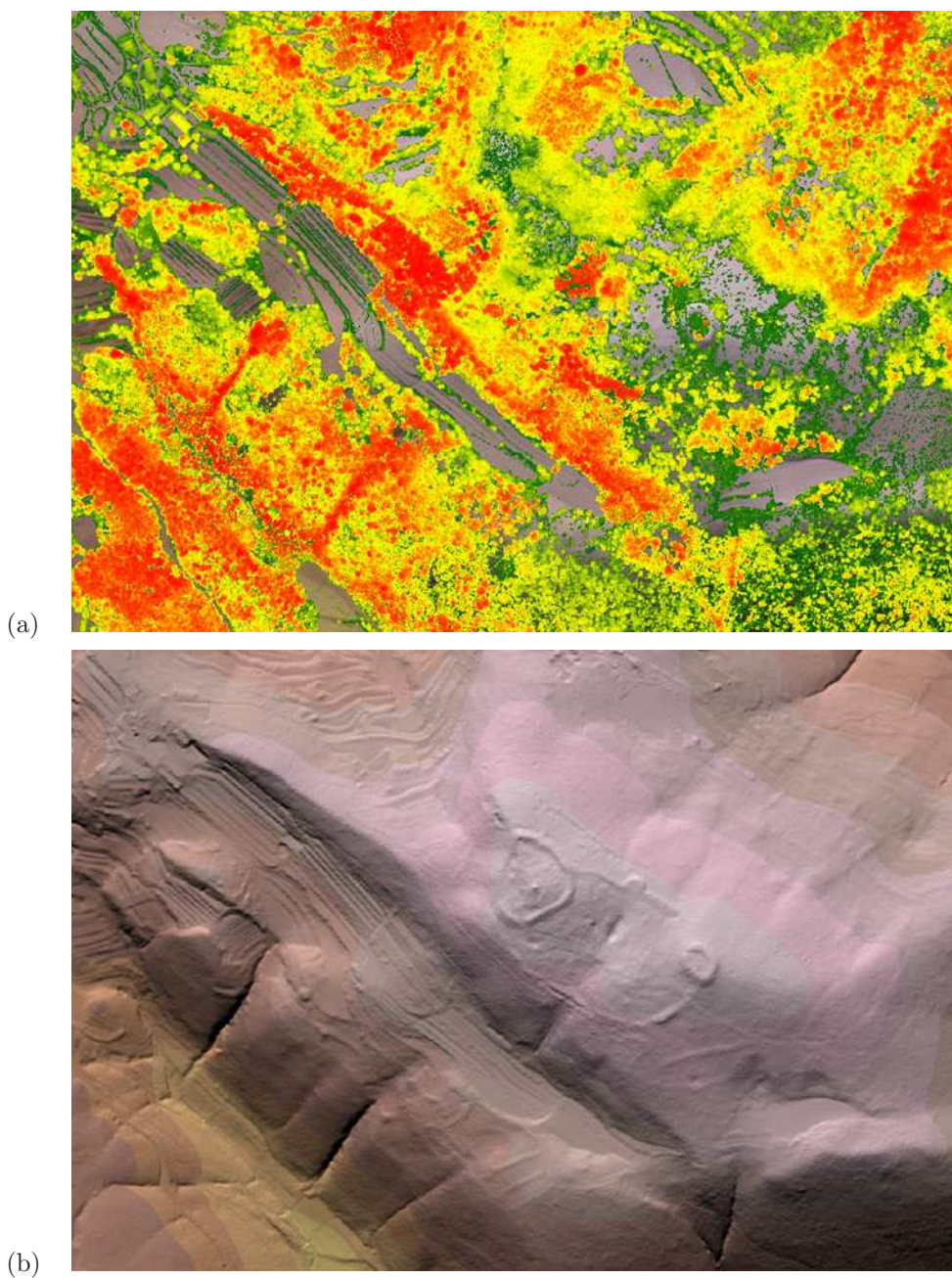
Slika 20.5: Lidar omogoča opazovanje podrobnosti pod drevesnimi krošnjami. Primerjava digitalnega modela višin, ki vključuje vegetacijski pokrov (a) in modela golih tal (b) razkriva arheološko najdišče, ki ga na letalskih fotografijah ne opazimo, saj ga zakriva bujno drevesje (Kobler et al., 2006).
