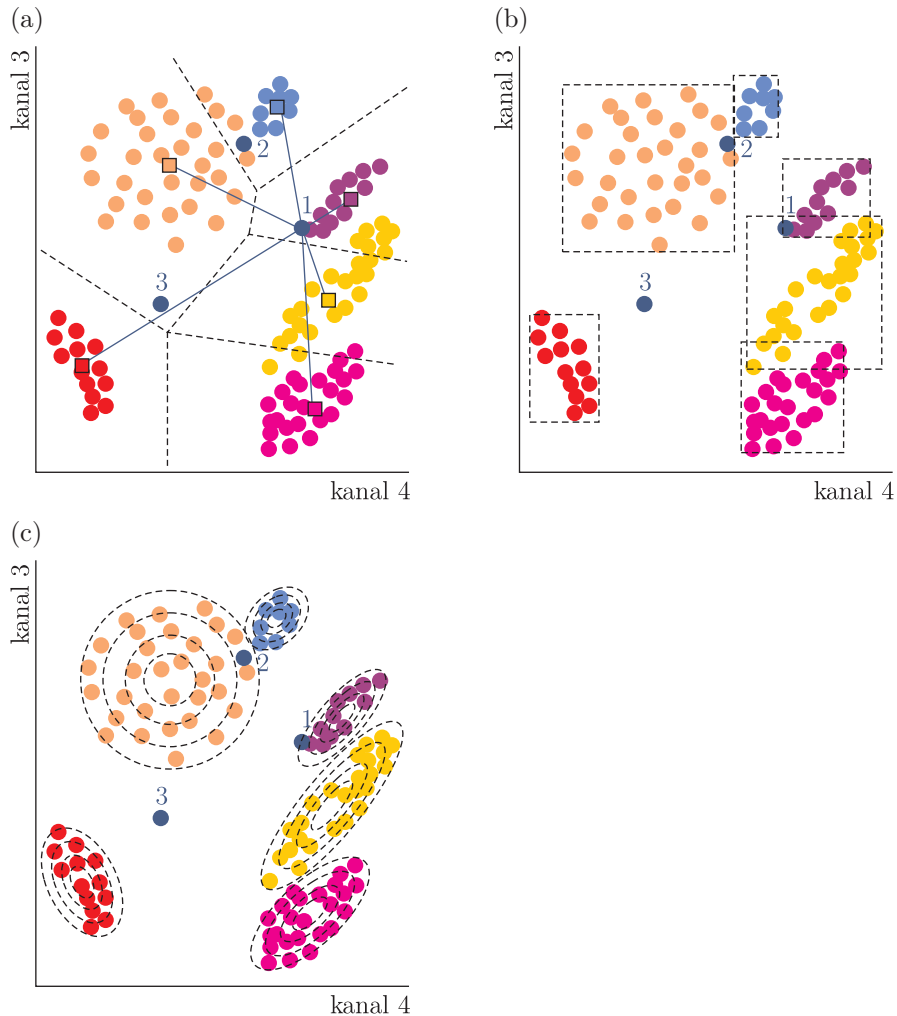
Slika 18.4: Pri klasifikaciji uporabljamo več različnih algoritmov, na primer metodo najmanjše razdalje (a), paralelepipedno metodo (b) ali metodo največje verjetnosti (c).
