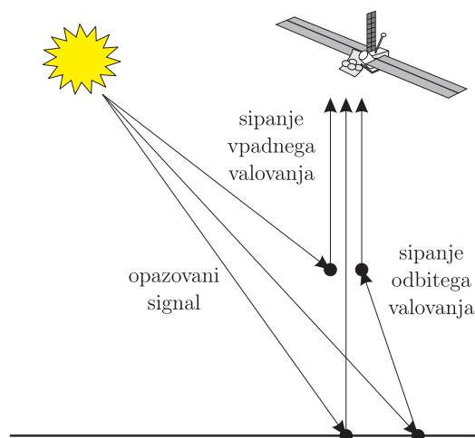
Slika 15.5: Na signal, ki ga zazna detektor, vplivajo različna vpadna valovanja.
