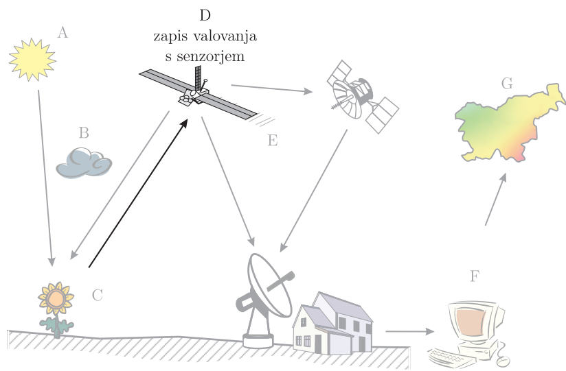
Slika 6.1: Zapis elektromagnetnega valovanja s senzorjem.
