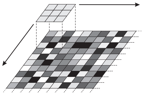
Slika 16.12: Pri konvolucijskem filtriranju prek podobe pošljemo računsko okno in v njem izvedemo določeno operacijo.
