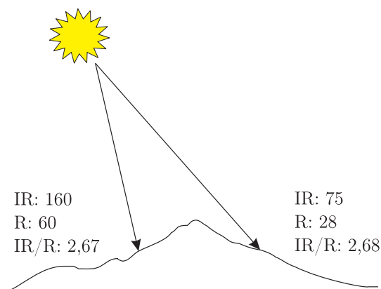
Slika 17.3: Razmerje kanalov je zelo podobno na osvetljenem in na senčnem delu podobe, kljub temu da so vrednosti v posameznih kanalih zelo različne.
