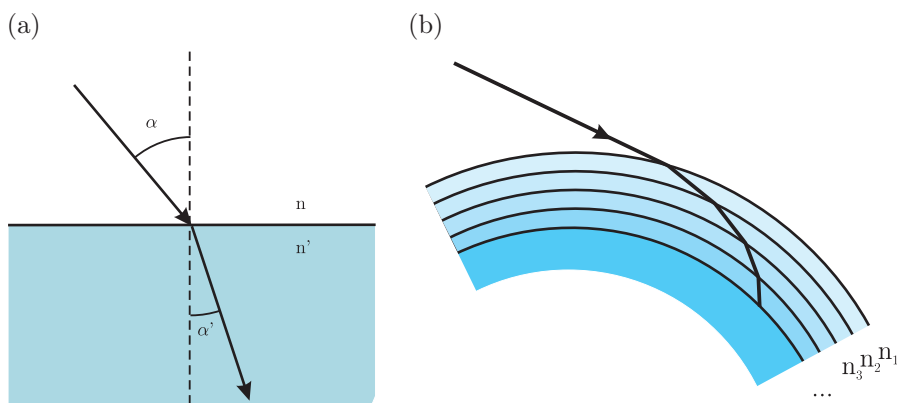
Slika 4.6: Lom svetlobe pri prehodu iz optično redkejši snovi v optično gostejšo (a) in potovanje žarka svetlobe skozi atmosfero (b).
