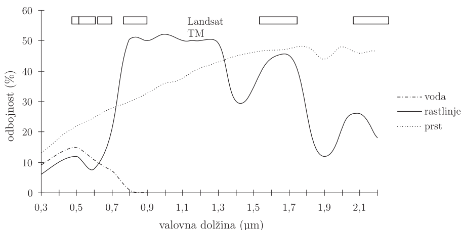
Slika 18.1: Spektralni podpis različnih tipov tal (vode, prsti in vegetacije). Označeni so tudi kanali senzorja Landsat Thematic Mapper.
